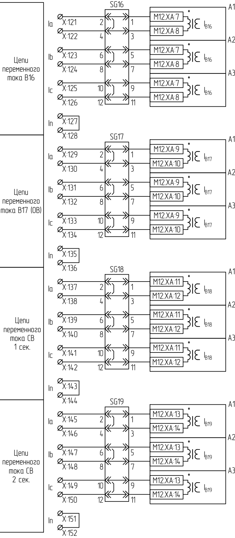
Цепи переменного тока
